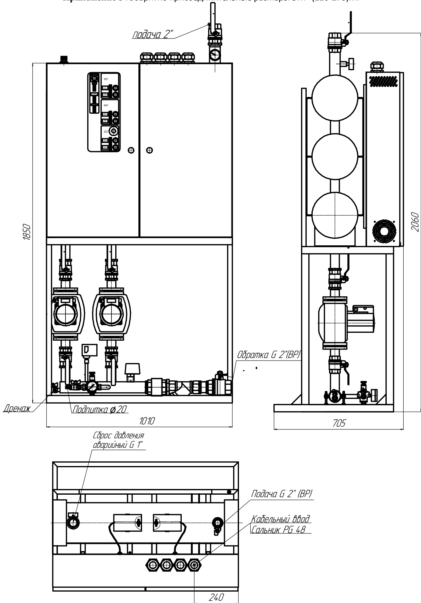
Габаритно-присоединительные размеры ЭКТ-(210-270)МР
