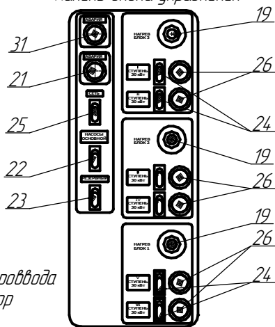
Панель блока управления
