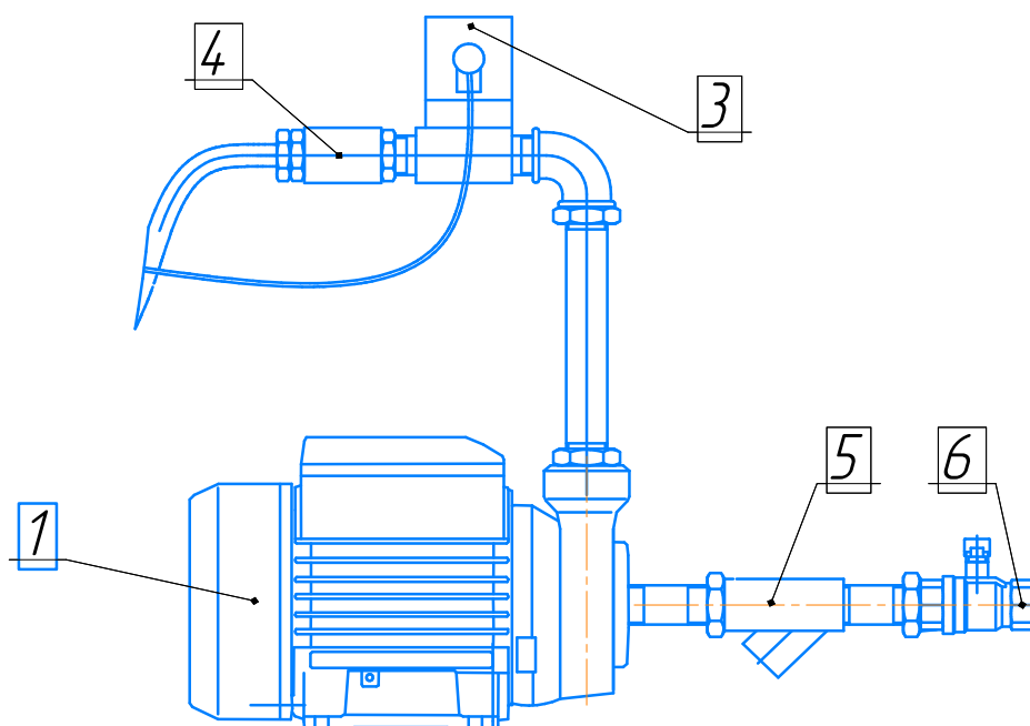
Рисунок 2: Система водоподготовки котла.
